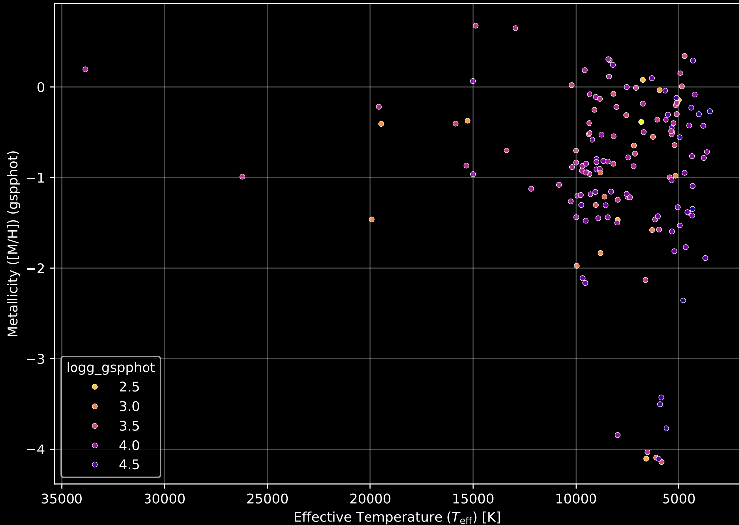
APOGEE DR17 Field: [160-60-C] Stellar Population Parameters (n= 148)
